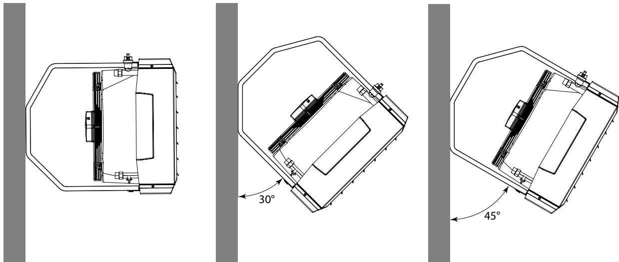
Figura 3.4 Posizionamento ventilante rispetto alla parete
