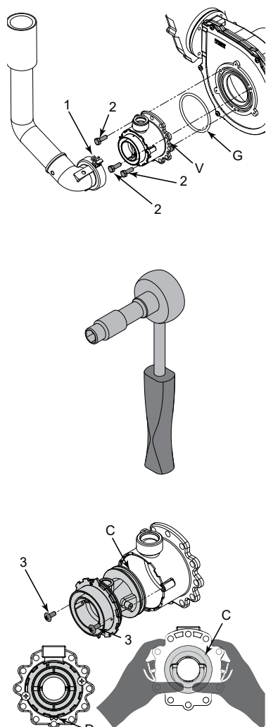
Figura 5.7 Cambio gas
