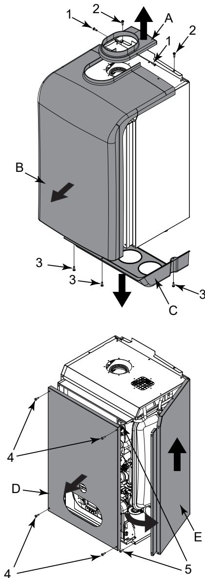
Figura 5.1 Accesso caldaia
