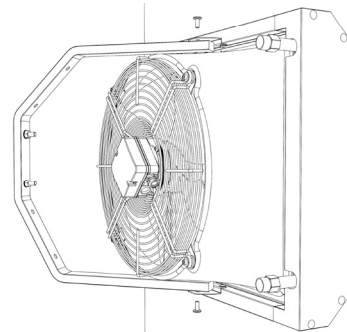
Figura 3.3 Fissaggio staffa alla ventilante
