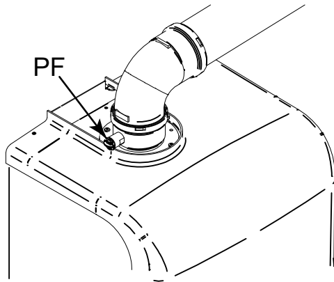
Figura 5.6 Presa fumi e valvola gas
