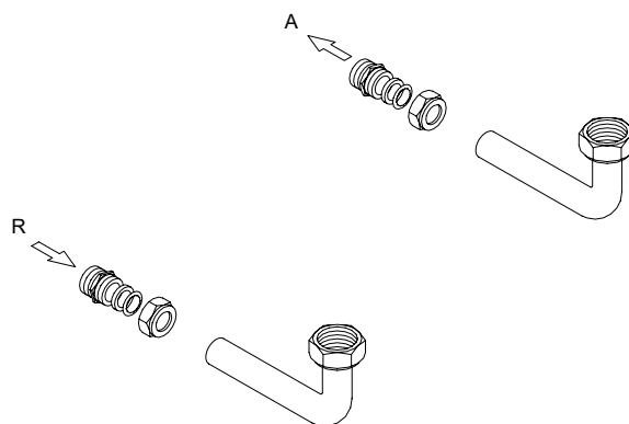
Figura 3.6 Kit raccordi idronici
