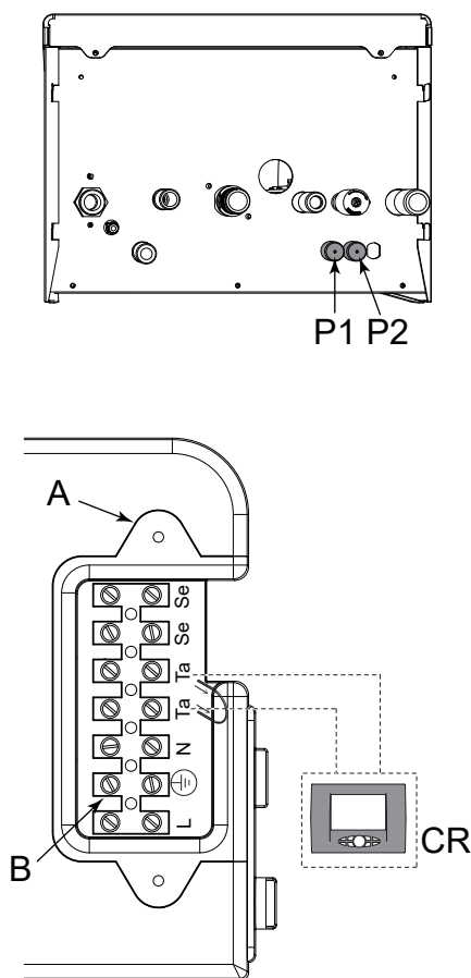
Figura 4.2 Posizione passacavi e dettaglio collegamento comando remoto al modulo esterno
