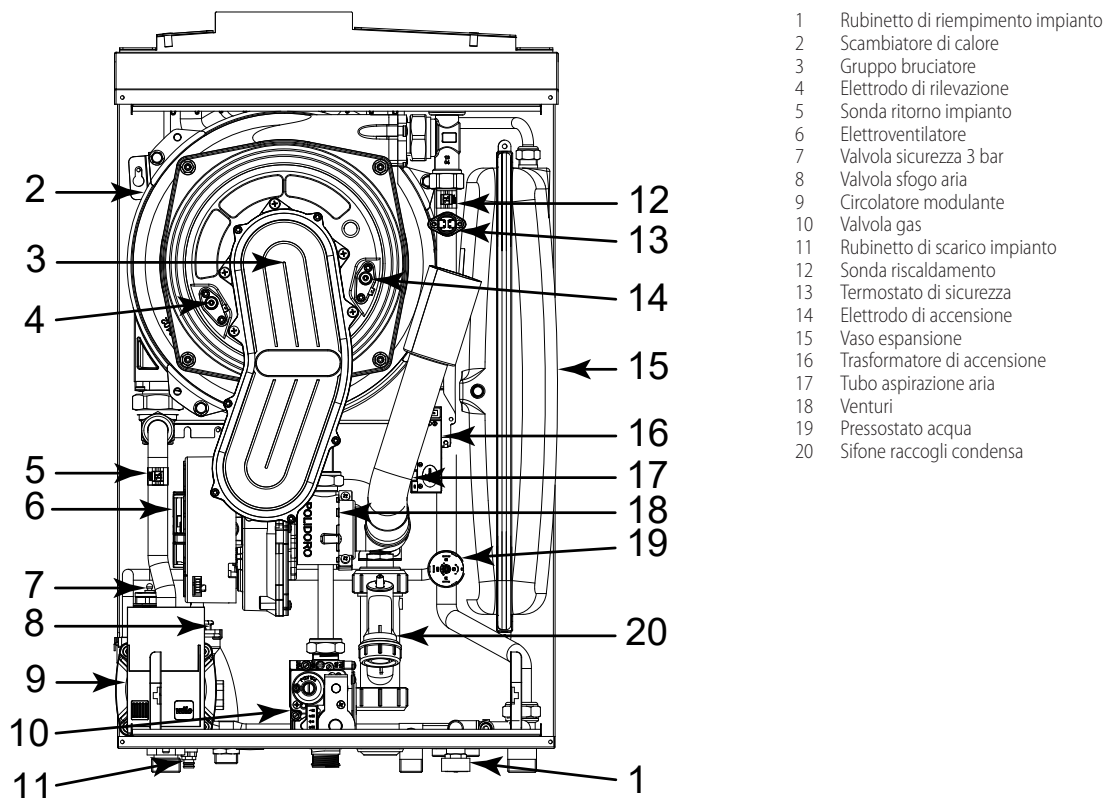
Figura 1.3 Vista frontale interna caldaia
