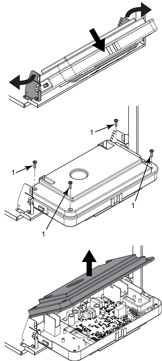
Figura 5.2 Accesso pannello comandi
