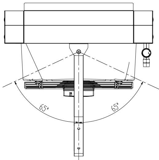
Figura 3.5 Orientamento ventilante
