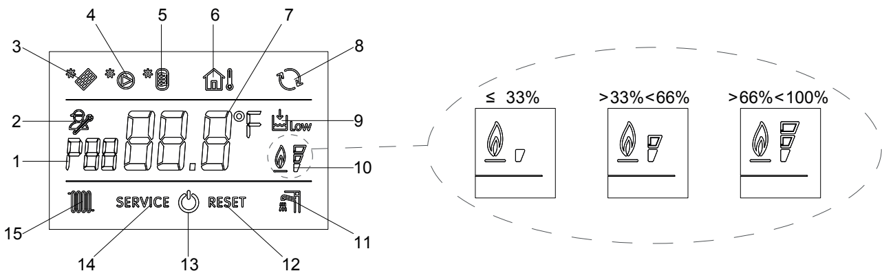
Figura 6.2 Icone Display caldaia
