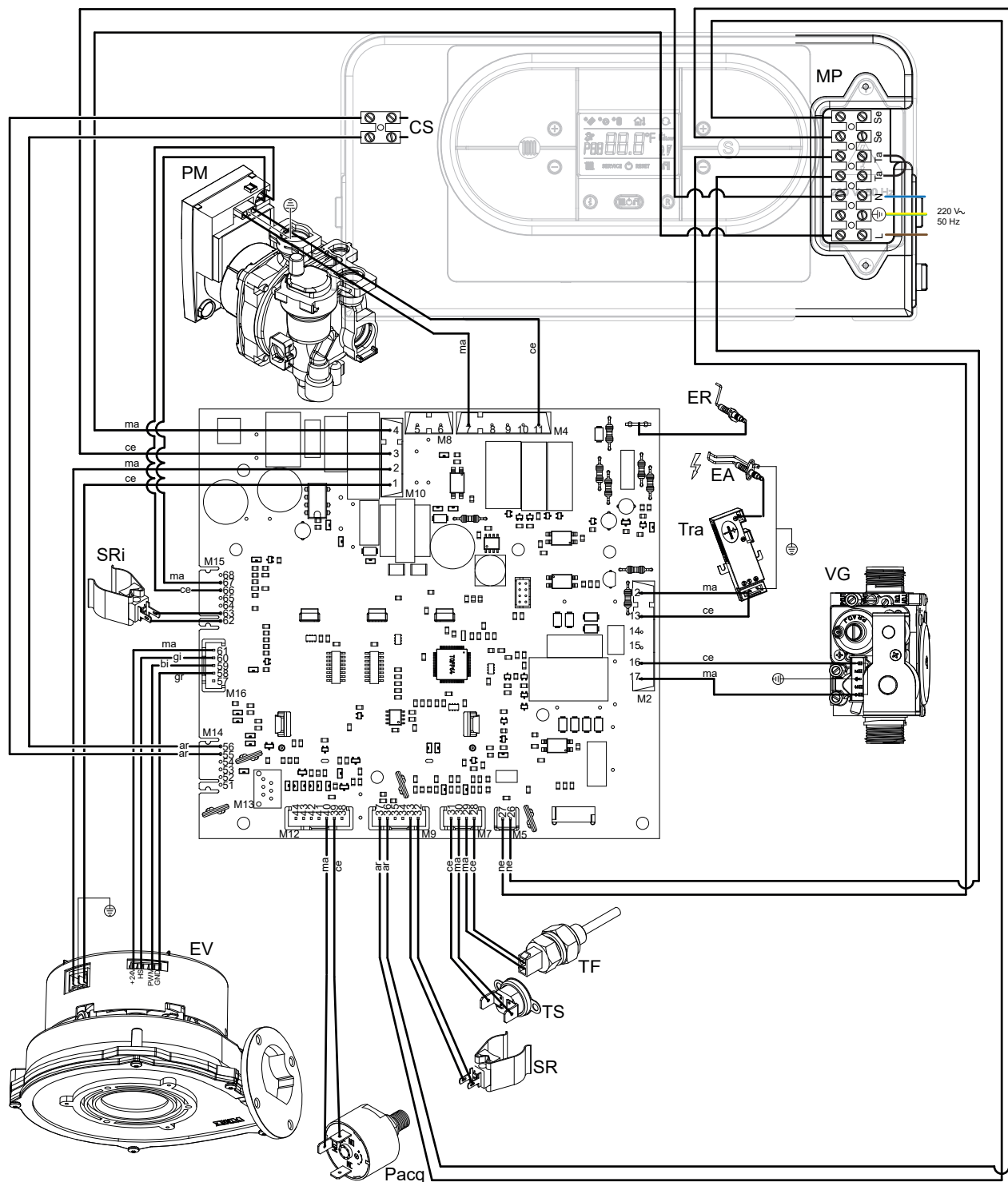
Figura 1.5 Quadro elettrico caldaia
