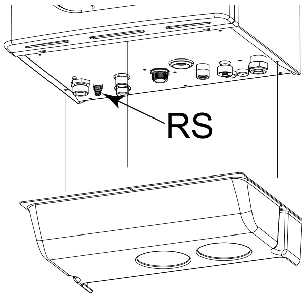
Figura 7.1 Posizione rubinetto di scarico impianto
