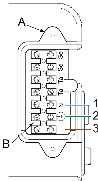
Figura 4.1 Alimentazione elettrica
