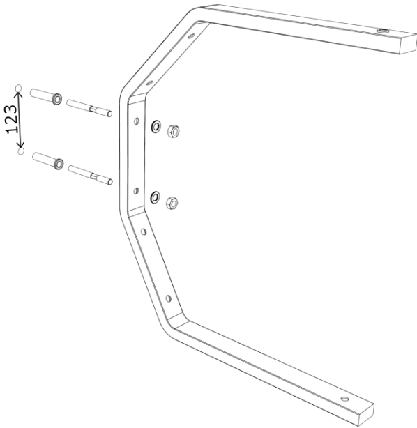
Figura 3.2 Posizione fori ventilante
