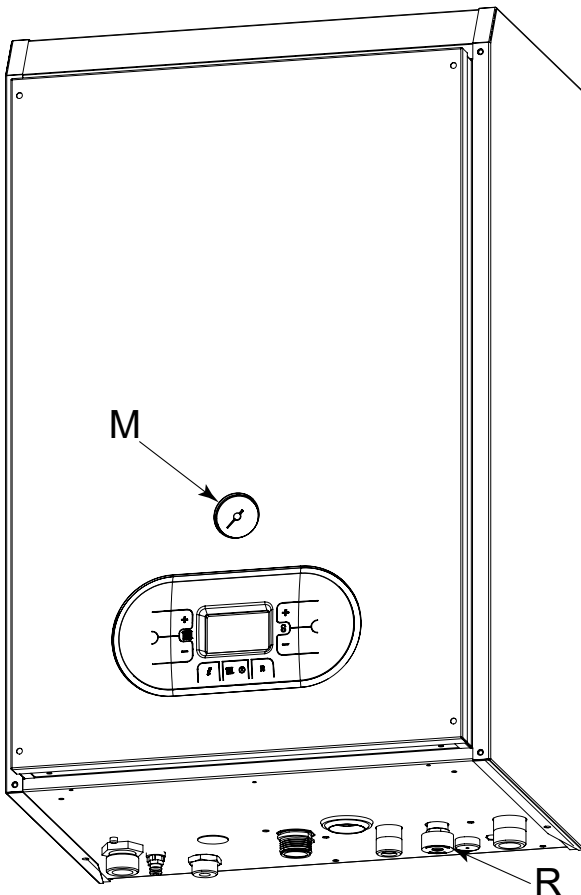
Figura 3.8 Manometro e rubinetto di carico impianto
