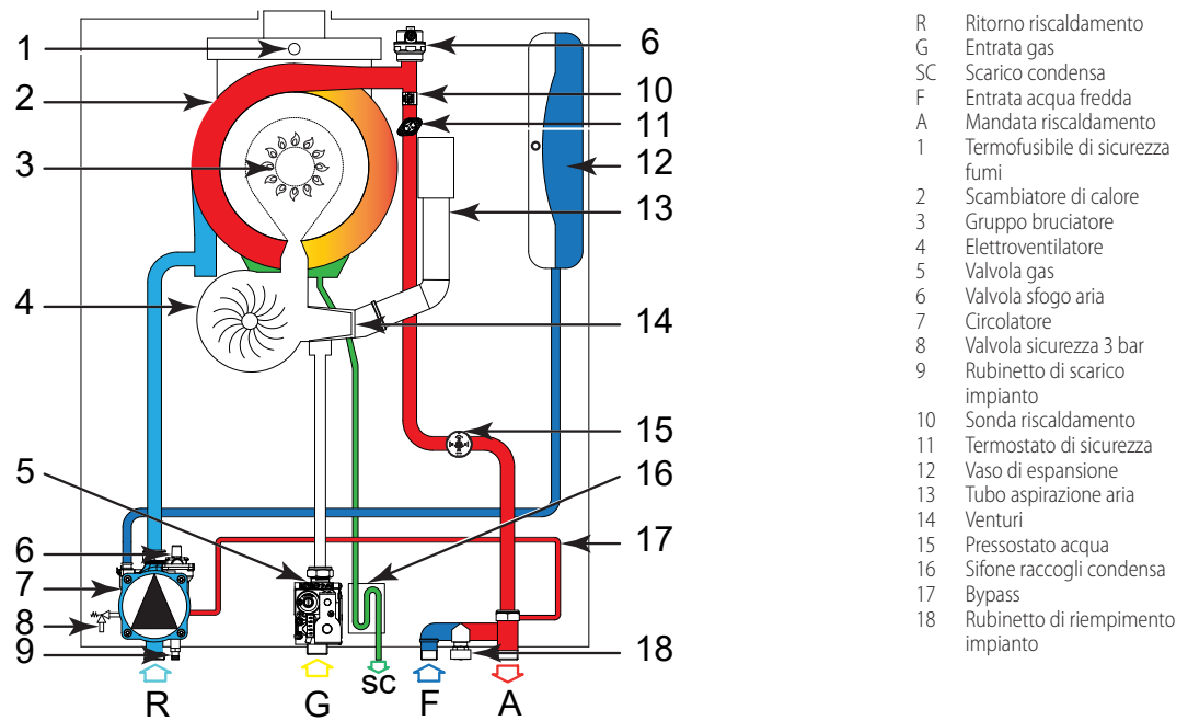
Figura 1.4 Schema idraulico interno caldaia
