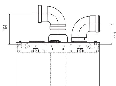
CONDOTTI SDOPPIATI PER SCARICO FUMI/ASPIRAZIONE ARIA
